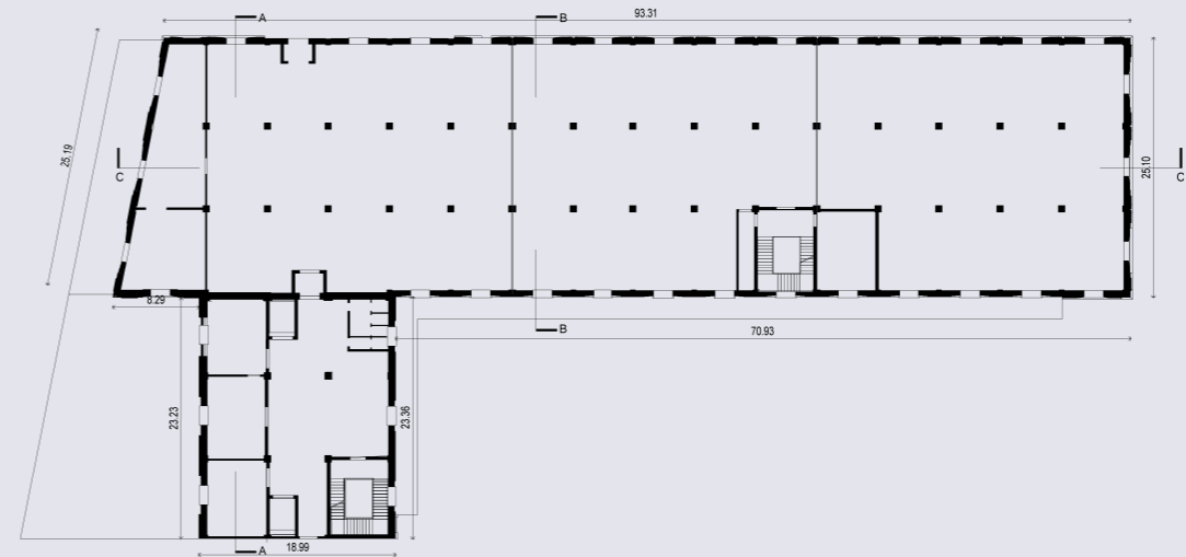
PIANTA LIVELLO 1
