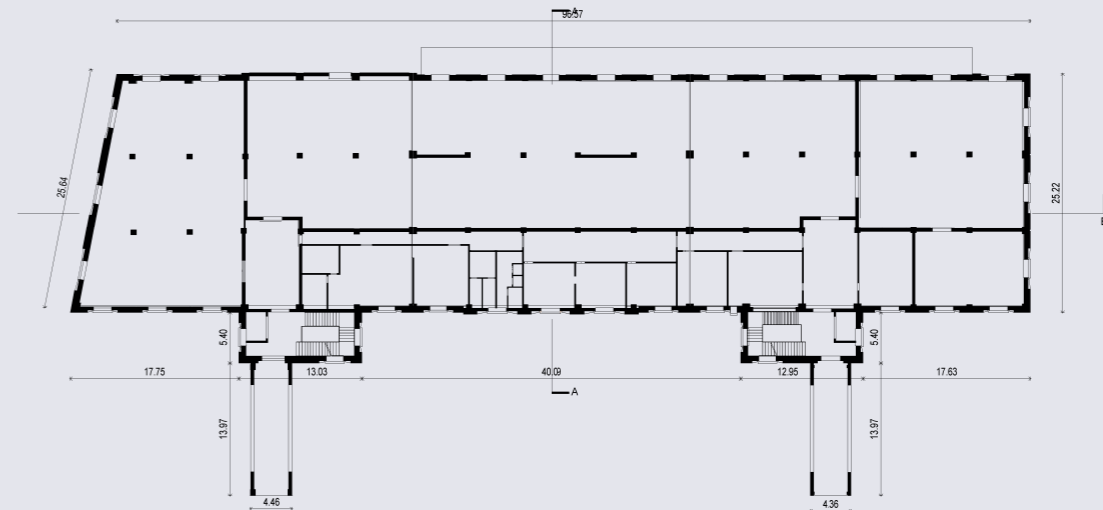
PIANTA LIVELLO 1
