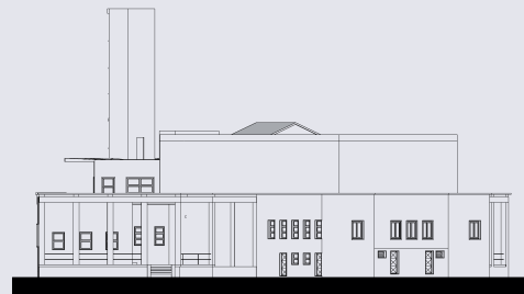
PROSPETTO OVEST
