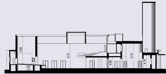
SEZIONE AA
