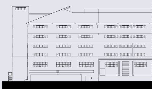
PROSPETTO SUD
