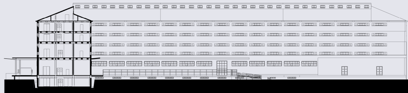
PROSPETTO EST
