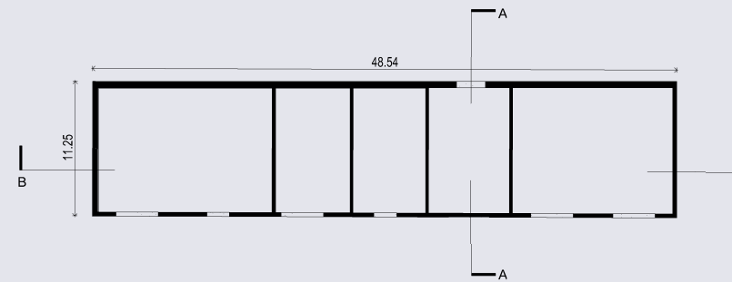
PIANTA LIVELLO 0
